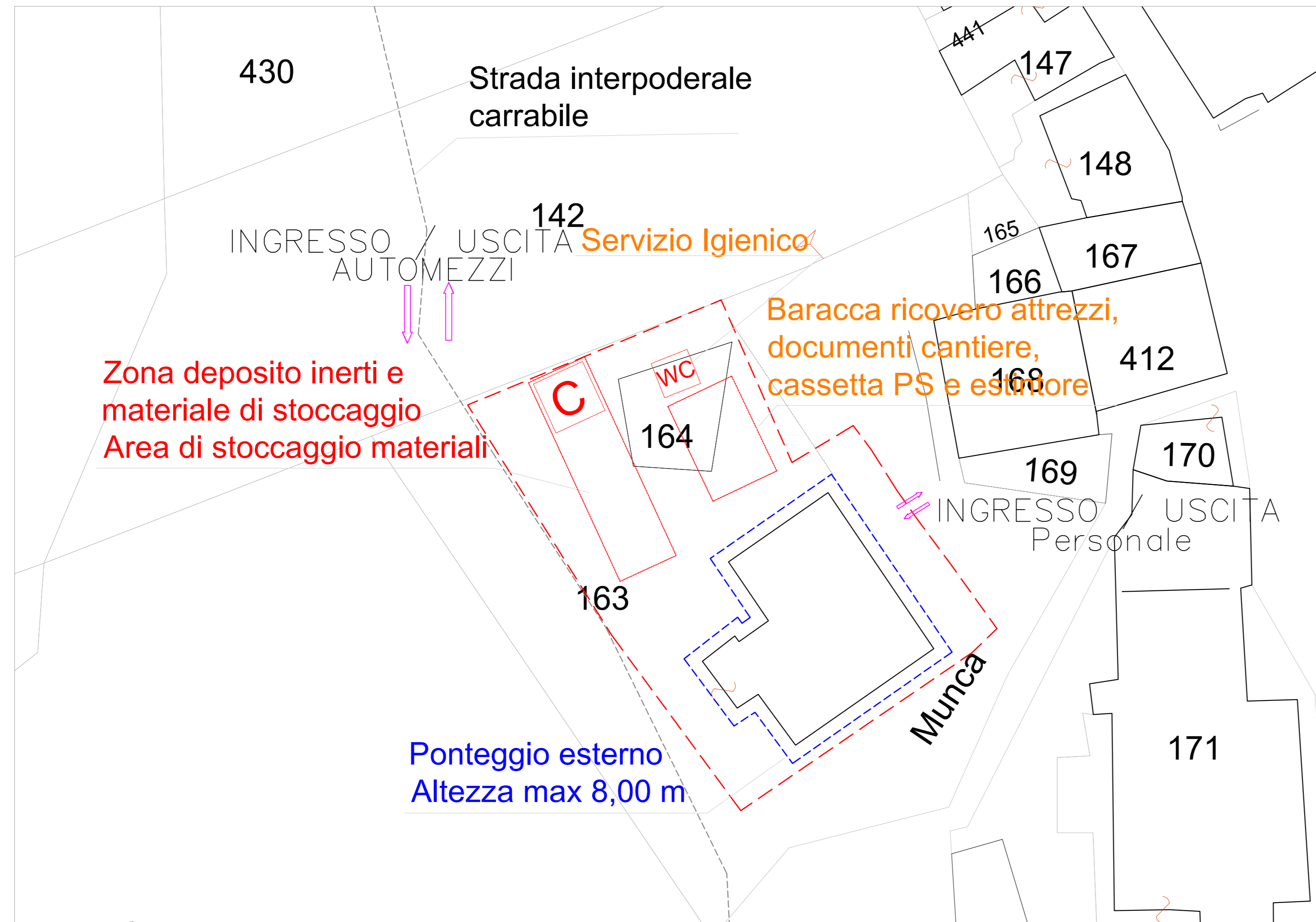
Layout di cantiere - Scala 1:250
