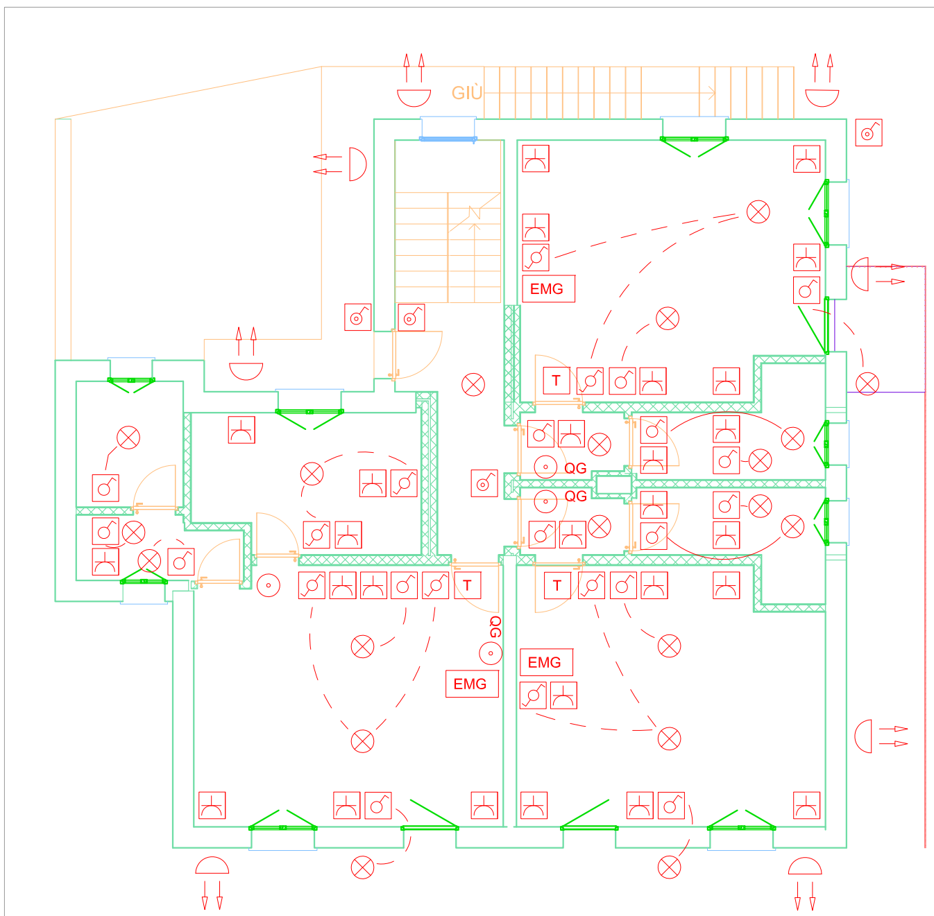
Impianto Elettrico - Piano primo - Scala 1:100
