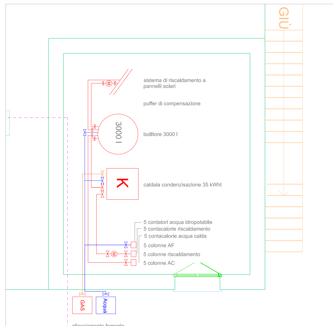
Impianto Termoidraulico - Piano terra - Scala 1:100
