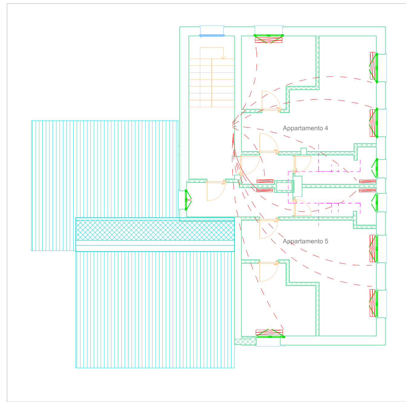
Impianto Termoidraulico - Piano secondo - Scala 1:100
