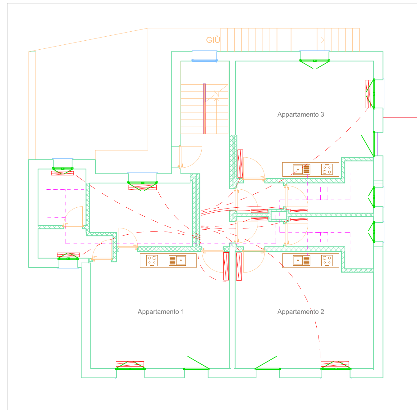
Impianto Termoidraulico - Piano primo - Scala 1:100
