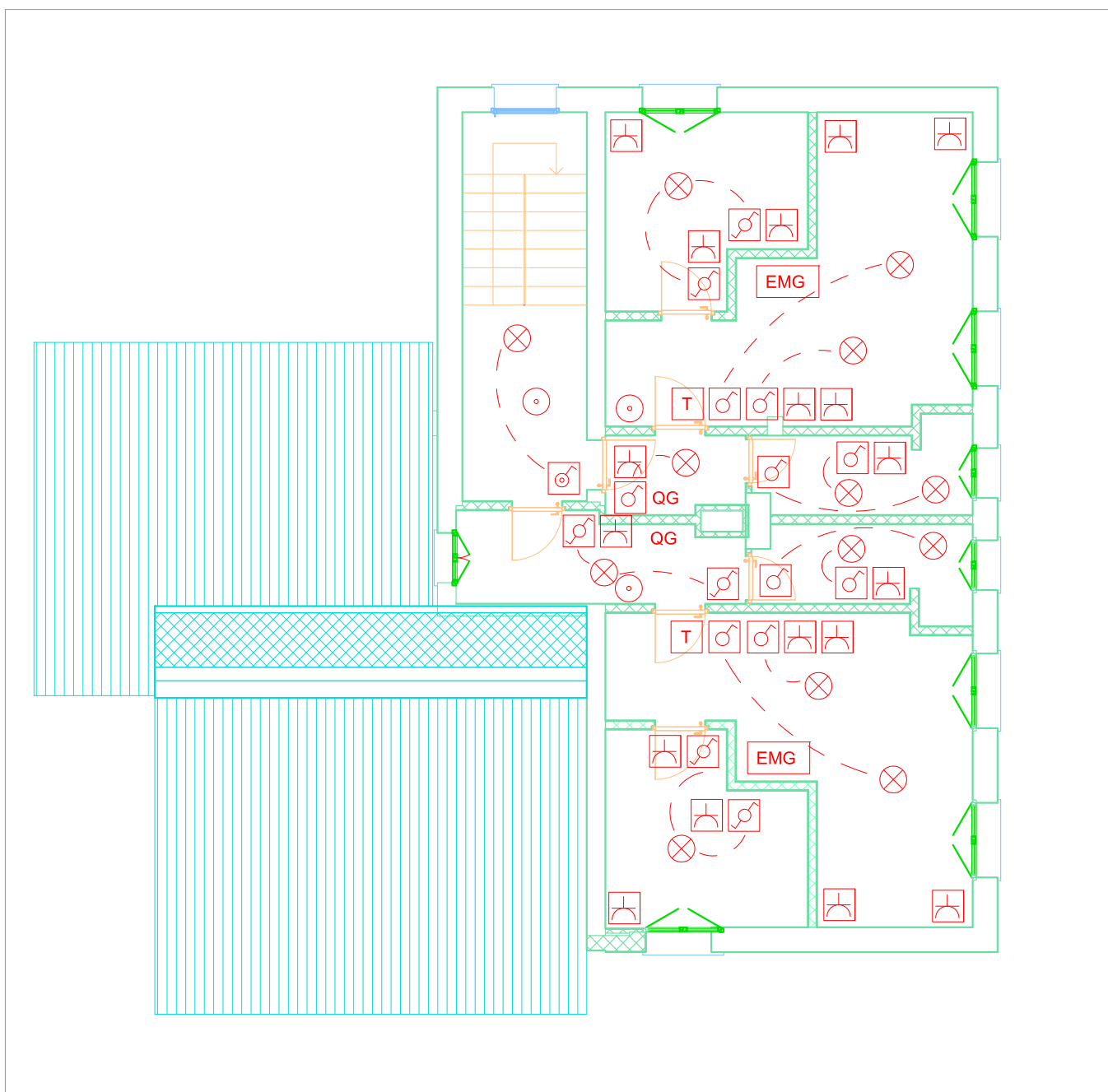
Impianto Elettrico - Piano secondo - Scala 1:100
