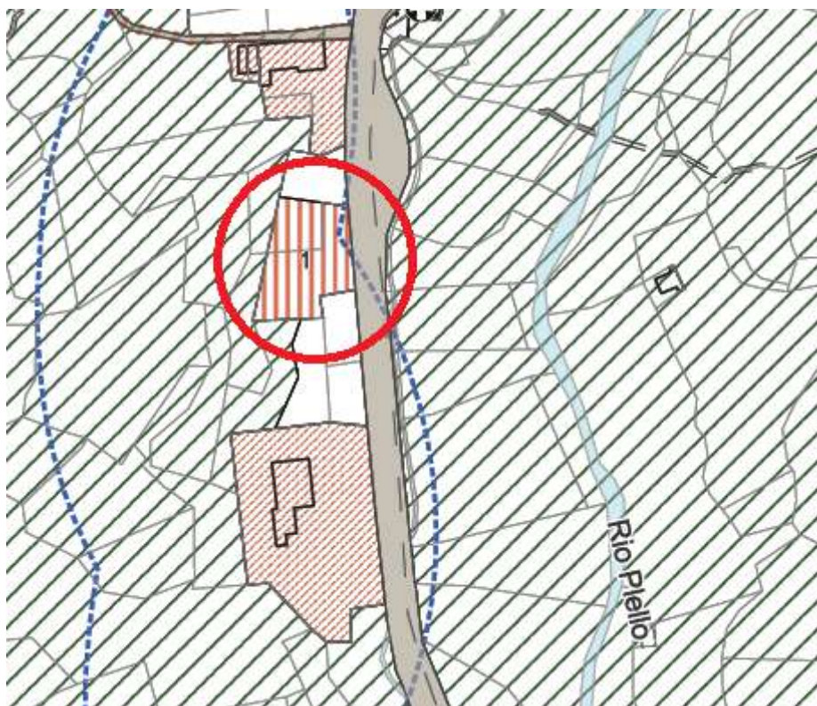
ESTRATTO DA ELABORATO SERIE 3P DELLA PROPOSTA TECNICA PROGETTO DEFINITIVO
